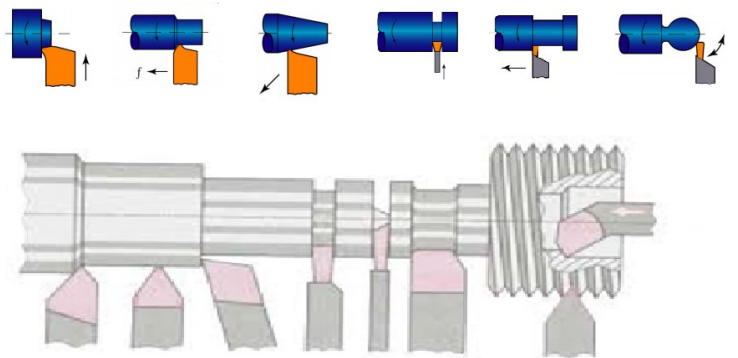
Şekil 1. Tornalama İşlemleri
