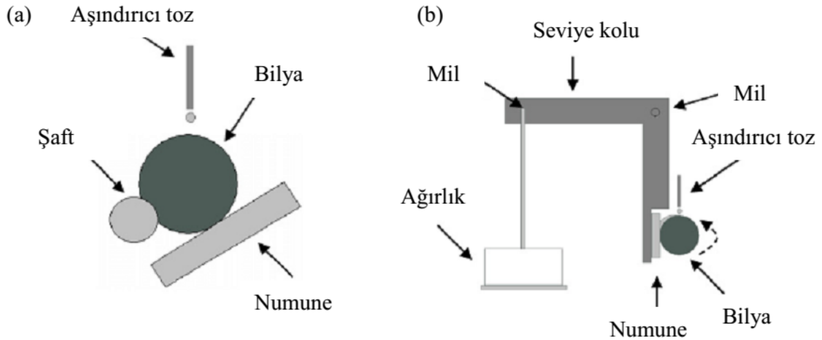
Şekil 5 Mikro abrazyon aşınma testi şeması
