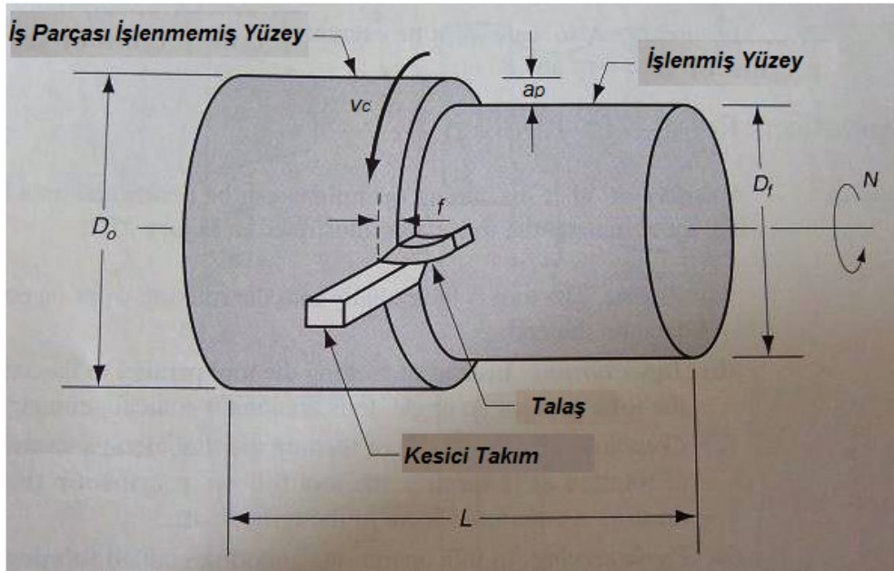
Şekil 2. Silindirik tornalama
