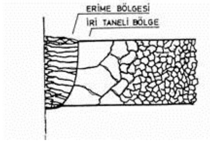
Şekil 2. ITAB’de tanelerin durumu (Şematik; Dönüşüm yoluyla mukavemet kazandırılan alaşımlar)
